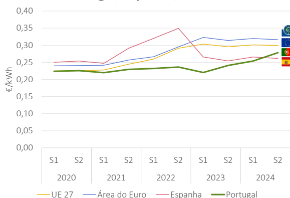
Figura 2 – Evolução de preços médios de eletricidade dos consumidores domésticos em Portugal, Espanha, UE e AE
