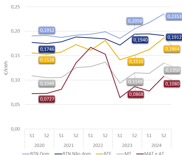
Figura 19 – Evolução dos preços médios por nível de tensão (sem IVA)
