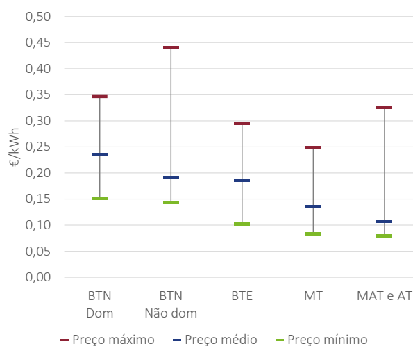
Figura 20 – Gama de preços (sem IVA) por nível de tensão
