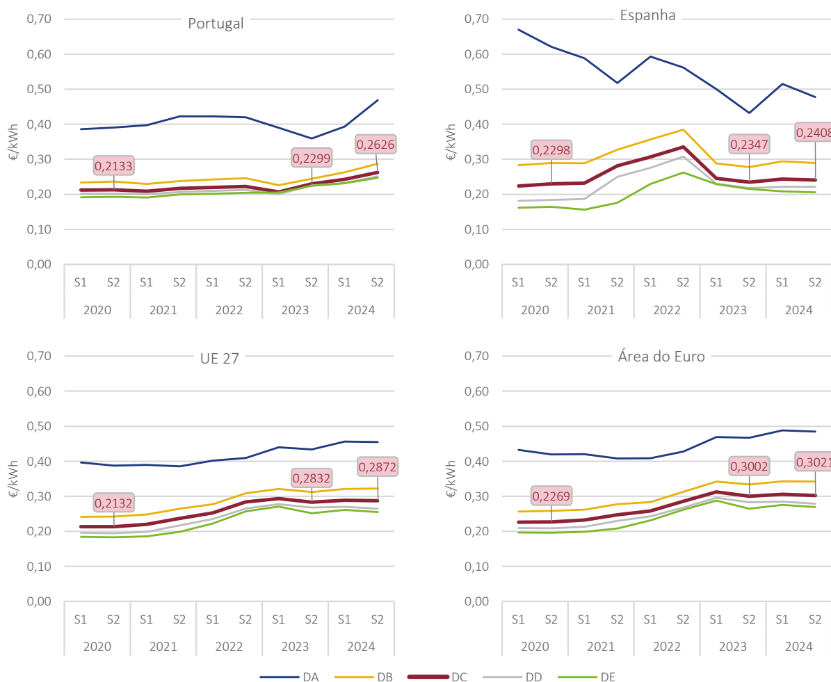
Figura 6 – Evolução de preços médios de eletricidade dos consumidores domésticos por banda de consumo Portugal, Espanha, União Europeia e Área do Euro
