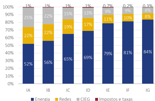
Figura 17 – Estrutura de preços médios de eletricidade - % (consumidores não domésticos)
